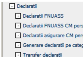
Figura 3.3-1 Meniul Declarații
